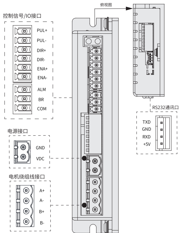
图 3-3 DM1 系列端子接口分布示意图
