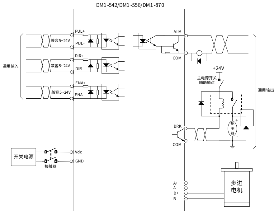
图 3-2 DM1 系列电气接线示意图
