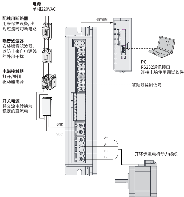
图 3-1 DM1 系列驱动器系统接线图
