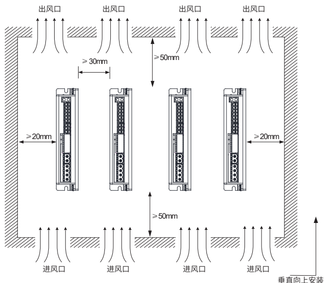
图 2-3 驱动器安装方式示意图
