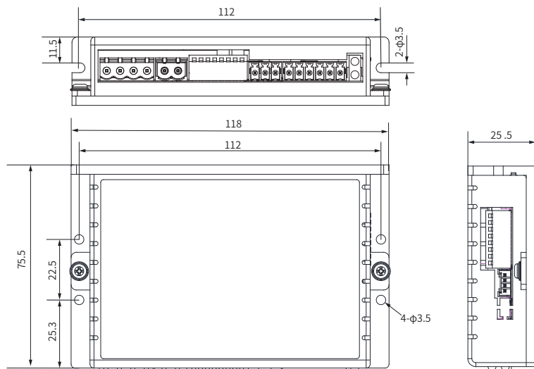
图 2-1 DM1-542 驱动器安装尺寸图 (单位: mm)
