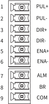
图 3-6 控制信号 /IO 端口示意图
